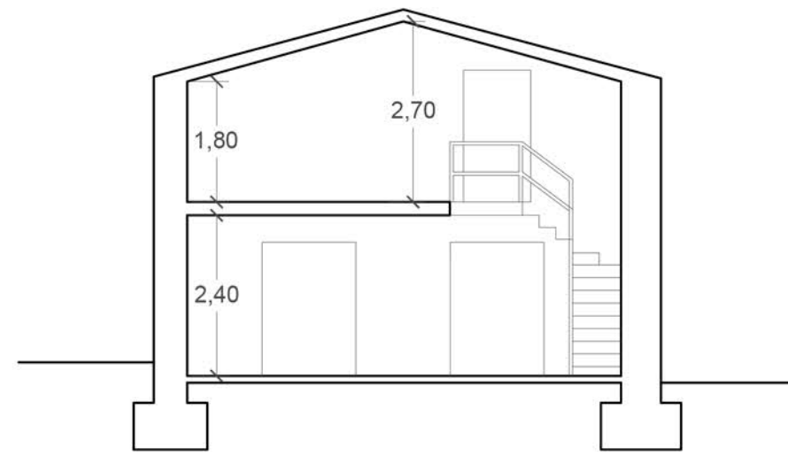
SEZIONE A-A
